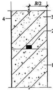
图 9.2.14-3 施工缝防水构造 (三)
