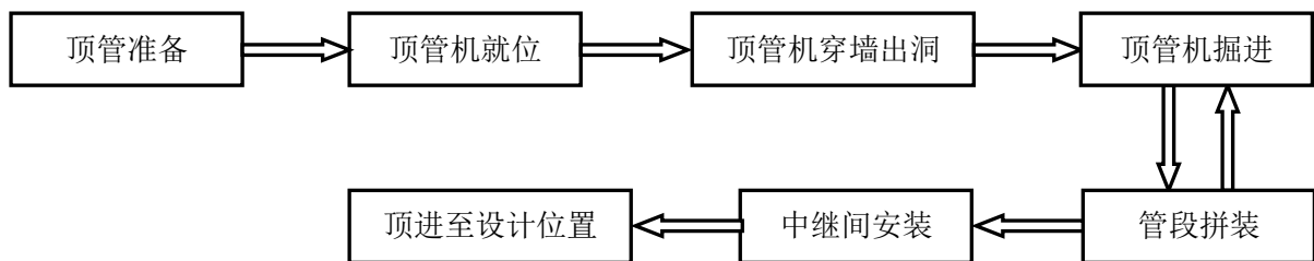
图 8.3.20 顶管施工流程图
