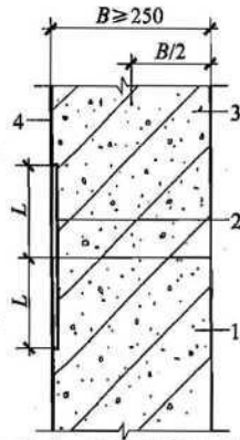
图 9.2.14-2 施工缝防水构造 (二)
