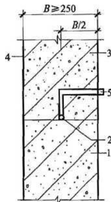
图 9.2.14-4 施工缝防水构造 (一)
